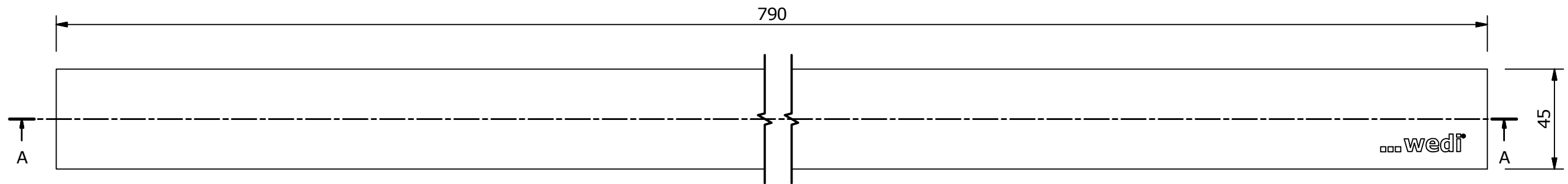
Draufsicht ( 1 : 2 )
