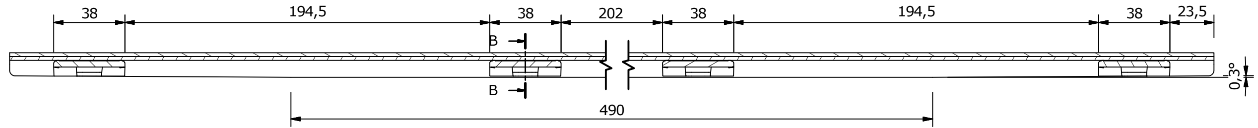
Schnitt A-A (1 : 2)
