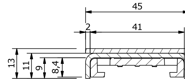
Schnitt B-B (1 : 1)
